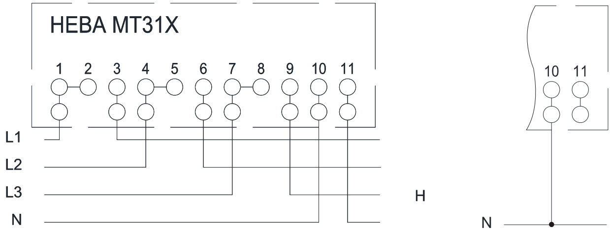
Схема включения счетчиков HEBA MT315 непосредственно в сеть
