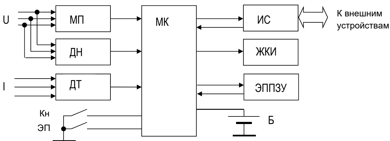
Рисунок 1.2 Функциональная схема счётчика.
