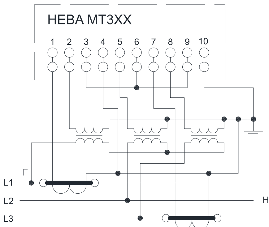
Схема включения счетчиков HEBA MT315 через два трансформатора тока и три трансформатора напряжения в трёхпроводную сеть
