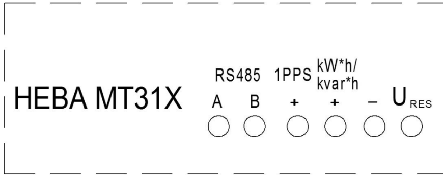
Схема подключения испытательных выходов счетчиков HEBA MT315 без промежуточного реле управления нагрузкой
