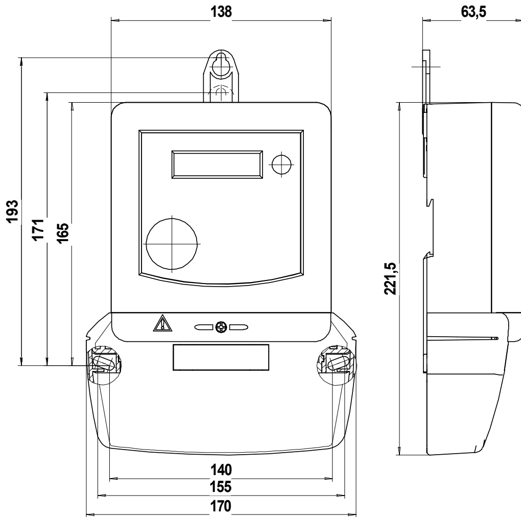
Внешний вид счетчиков НЕВА МТ315
