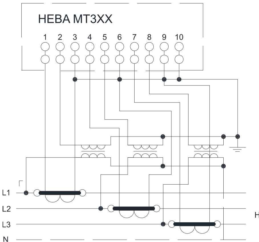
Схема включения счетчиков HEBA MT315 через трансформаторы тока и трансформаторы напряжения в трёх- и четырёхпроводную сеть.
