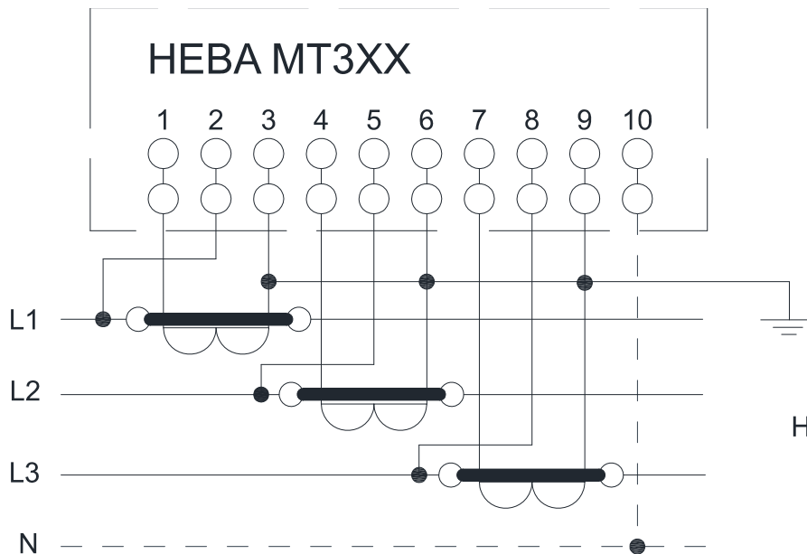
Схема включения счетчиков HEBA MT315 через трансформаторы тока в четырёхпроводную сеть
