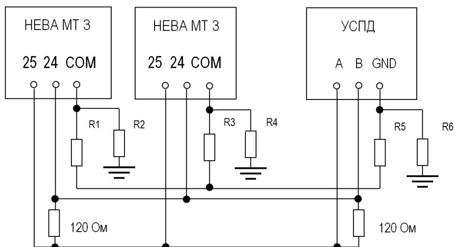
Рисунок 2.2 Схема подключения счётчиков к интерфейсной линии EIA 485
