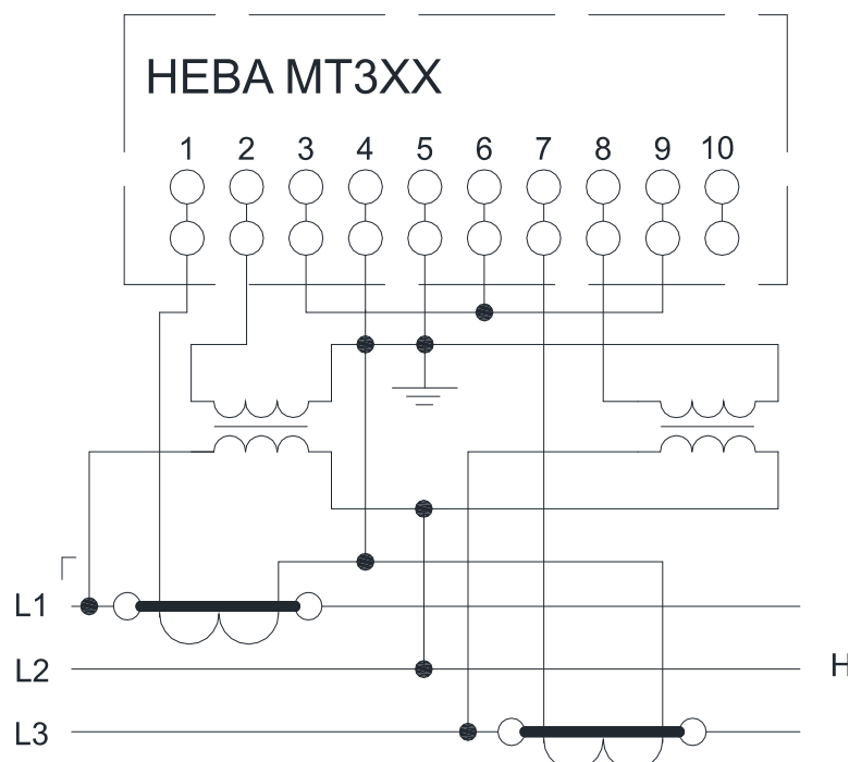
Схема включения счетчиков HEBA MT315 через трансформаторы тока и трансформаторы напряжения в трёхпроводную сеть
